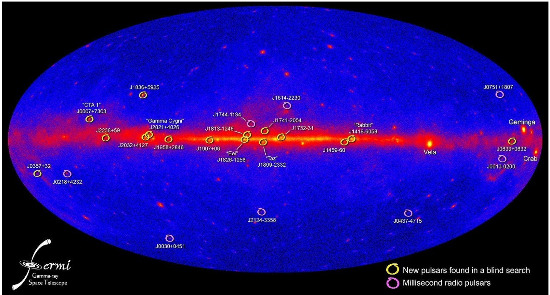
A Fermi által észlelt pulzárok eloszlása
