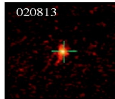
long GRBs
