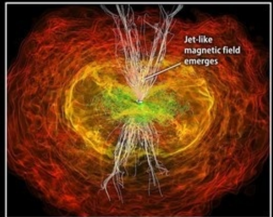
26.5 milliseconds
