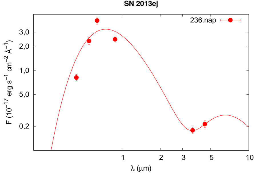
4. ábra. Az SN 2013ej 236. napjához tartozó, optikai fotometriai adatokkal kiegészített SED-jére illesztett forró modellkomponens.
