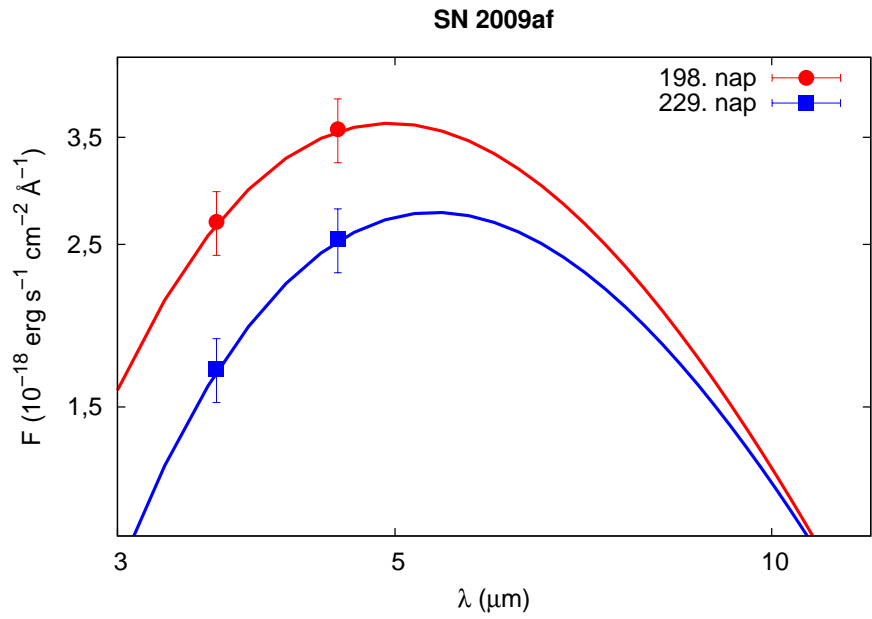
8. ábra. Az SN 2009af közép-infravörös SED-jei.
