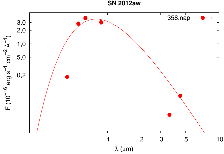
3. ábra. Az SN 2012aw 358. napjához tartozó, optikai fotometriai adatokkal kiegészített SED-jére illesztett forró modellkomponens.
