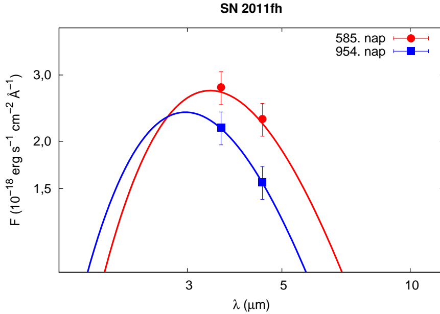
6. ábra. Az SN 2011fh közép-infravörös SED-jei.
