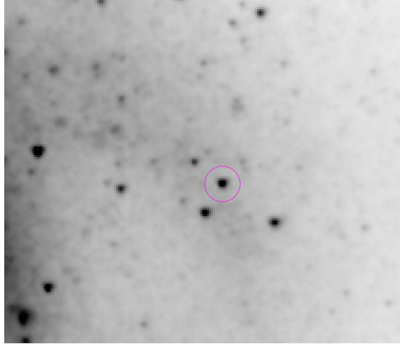
1. ábra. Egy az SN 2012aw-ról 3,6 \mu\text{m} -en készült Spitzer-felvétel.
